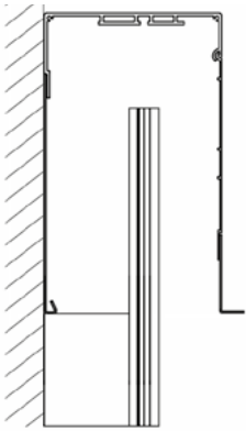
TYP A - Skrzynka pod zabudowę. Dedykowane prowadnice F-FBR-030.
