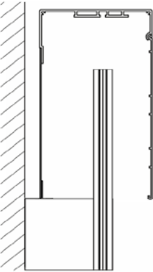
TYP D - Skrzynka na elewację z odsadzeniem. Dedykowane prowadnice F-FBR-020.
